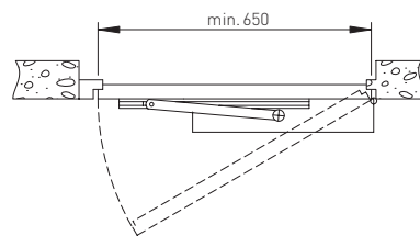
Плечо скользящего типа - SBS
