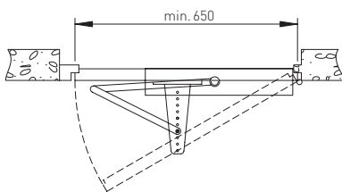
3х коленное плечо шарнирного типа - BRAS
