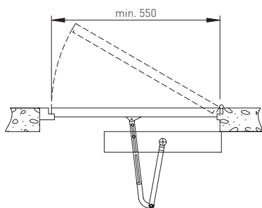
Плечо шарнирного типа - SBA
